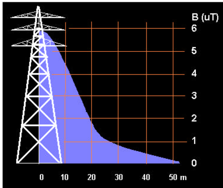
Figura 5. Valores de inducción magnética (en micorteslas, \mu\text{T} ) medidos a 1 metro de altura sobre el suelo, en las cercanías de una línea de transporte eléctrico (la torre no está representada a escala). Se observa que los valores de B se reducen significativamente al aumentar la distancia a la línea. Así, en la vertical de la línea, B podría alcanzar valores de hasta 6 \mu\text{T} ; a 15 metros de la línea, B se reduciría a la mitad, y para distancias superiores a 30 metros B estaría en el orden de las décimas del microtesla. El Consejo de Ministros de Sanidad de la Unión Europea recomienda que el público no esté expuesto a niveles de B superiores a 100 \mu\text{T}
